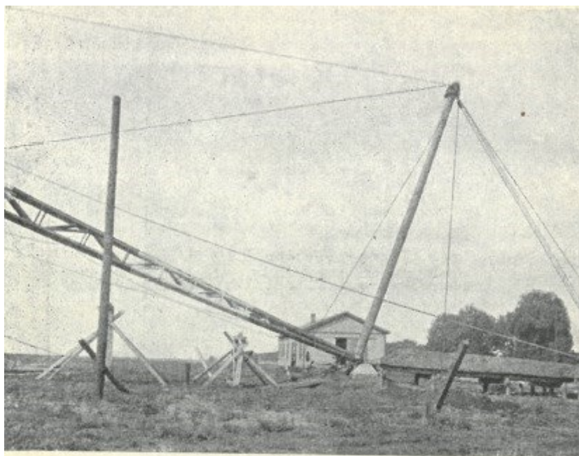
Vysílací stanice Kbely. Vztyčování stožáru.
