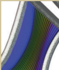
Expansion kinetic effect v paprscích insignie.
